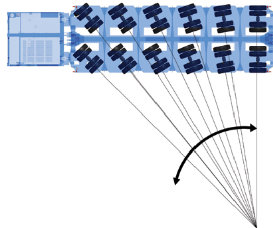
4. Vorderachslenkung
